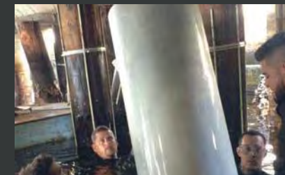
Chaqueta PileMedic® instalada antes de colocar el grout.
