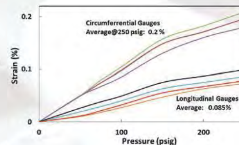
TENSIÓN CIRCUNFERENCIAL Y LONGITUDINAL
